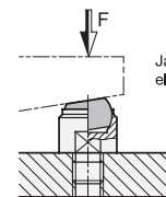
Przykład montażu
